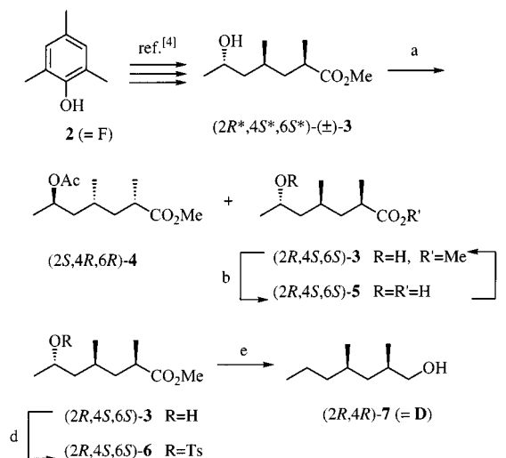
Scheme 3. Synthesis of the building block (2 R ,4 R )- 7 : reagents: (a) CH 2 =CHOAc, lipase AK, hexane [42% of (2 S ,4 R ,6 R )- 4 ; 46% of (2 R ,4 S ,6 S )- 3 ]; (b) LiOH, THF/H 2 O (99%), then recrystallization from Et 2 O/hexane (51%); (c) CH 2 N 2 , Et 2 O (99%); (d) TsCl, C 5 H 5 N (quant.); (e) LiAlH 4 , Et 2 O (83%)
